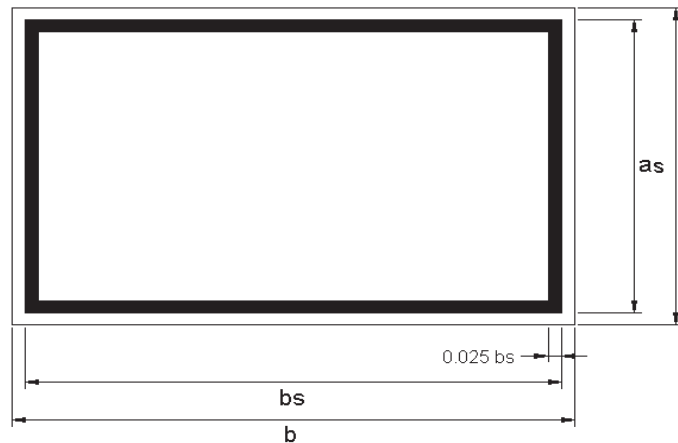
FIGURA 7 - Requisitos de diseño para información adicional enmarcada
